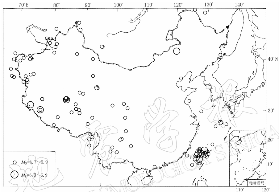
2004 年中国及邻区地震震中分布图
