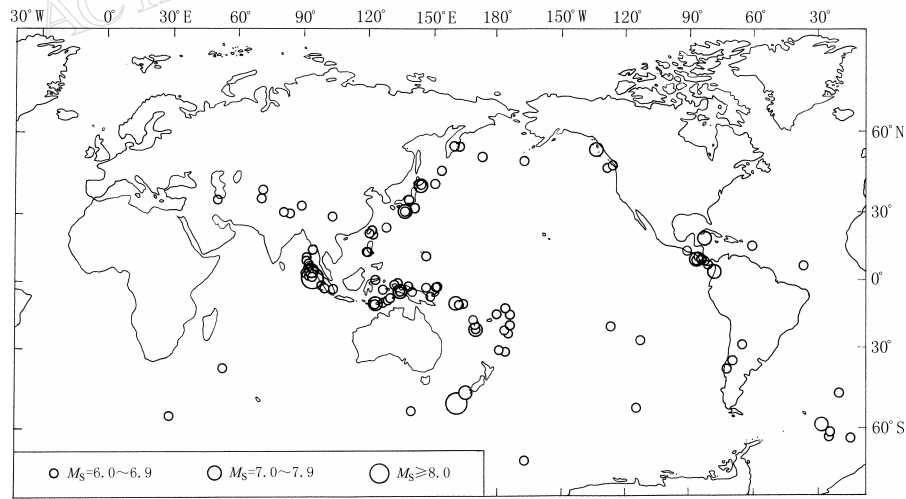
2004 年世界地震震中分布图
